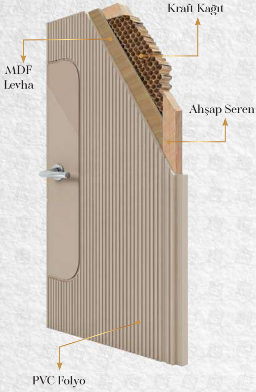
Membran Kapı İç Detayı
