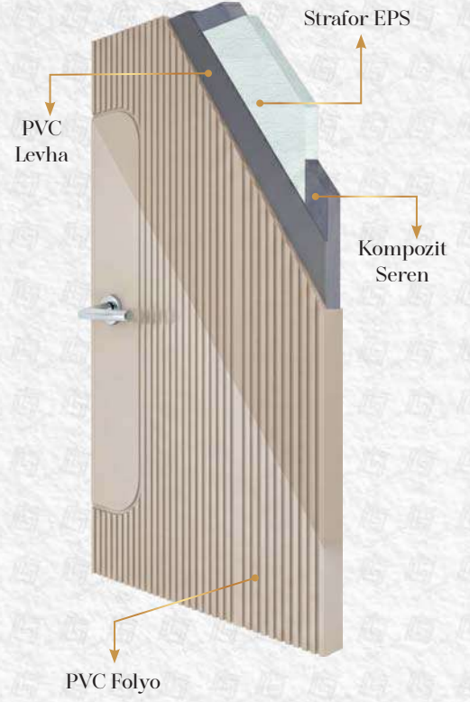
Kompozit Kapı İç Detayı
