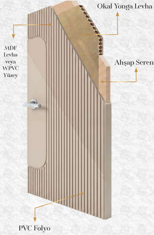
Opsiyonel Kapı İç Detayı
